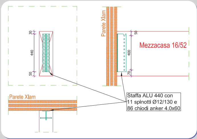
| Connessione Mezzacasa - Parete Xlam con staffa alu
