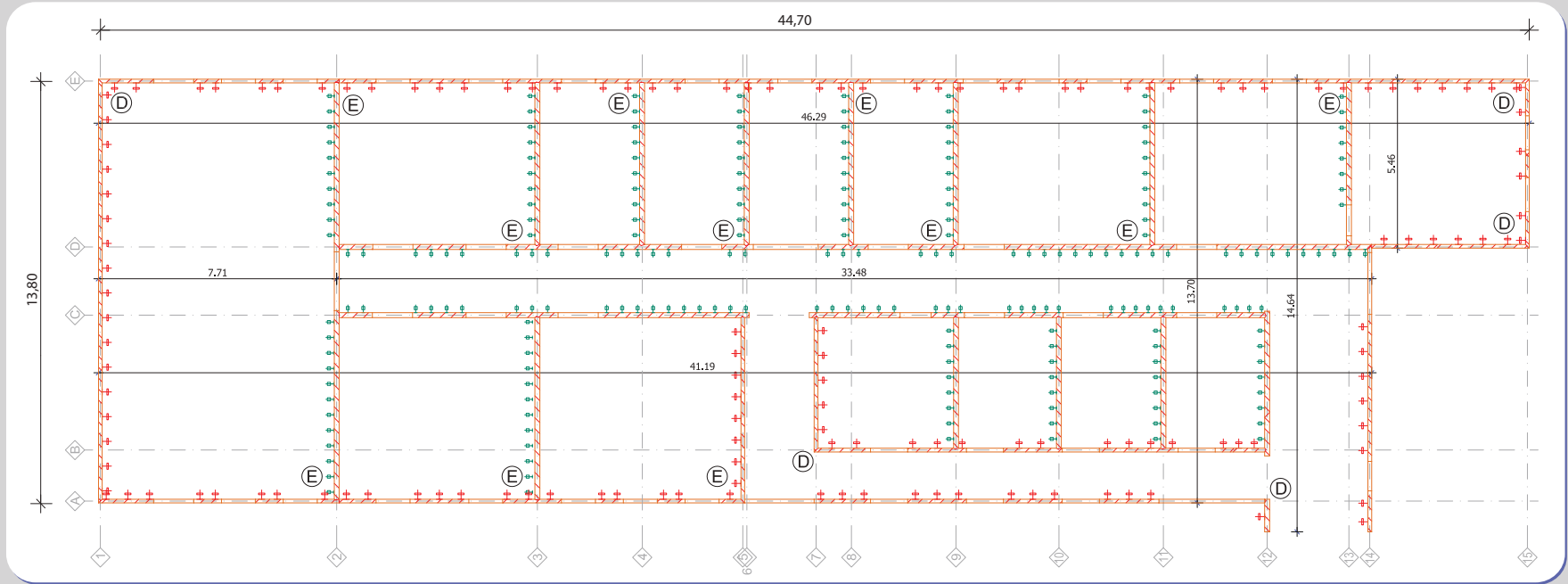
Pianta costruttivo Attacco a Terra
