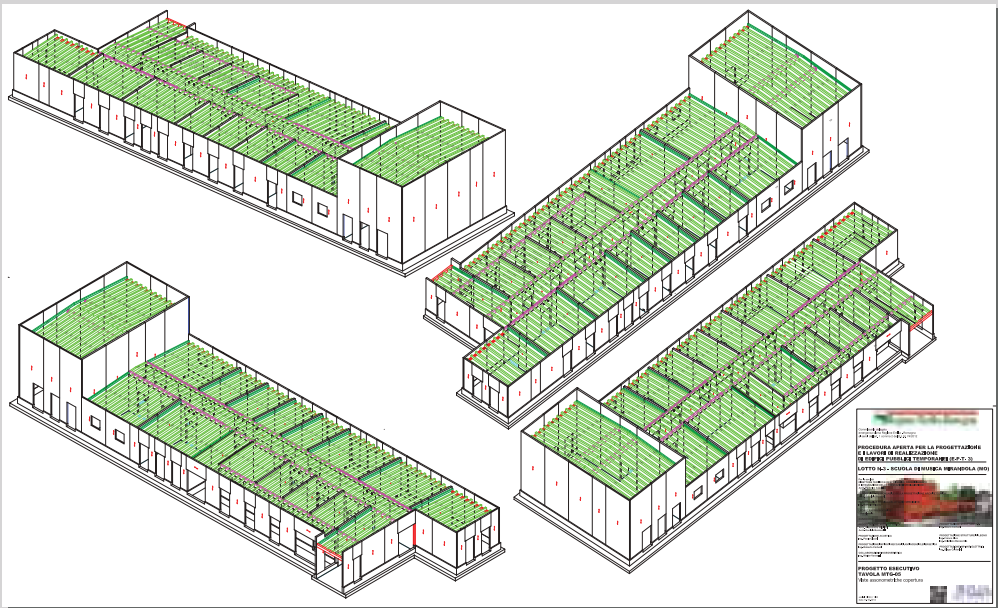
| Tavola di Montaggio Coperture dell'edificio
