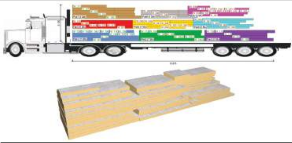
Piano di carico camion per trasporto pareti Xlam
