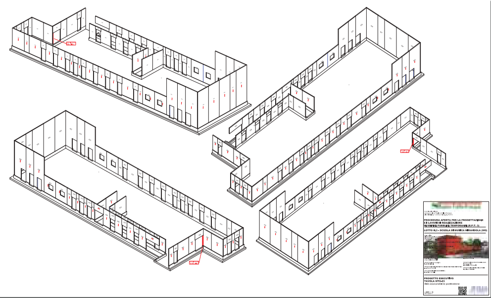
Tavola di Montaggio Pareti Xlam
