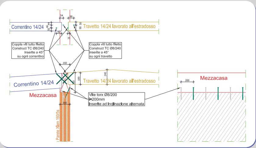
| Connessione delle diverse orditure di copertura alla mezzacasa
