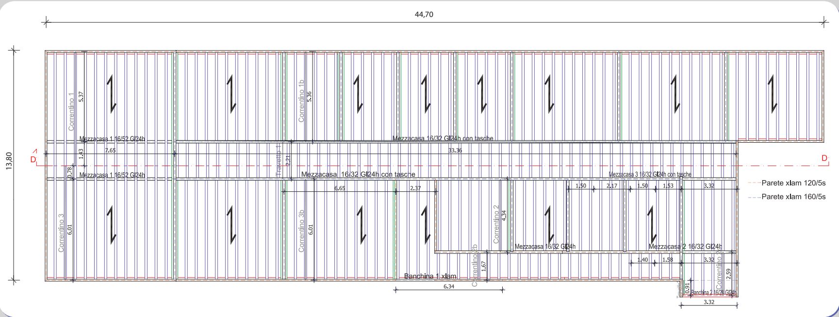
| Pianta costruttivo Copertura
